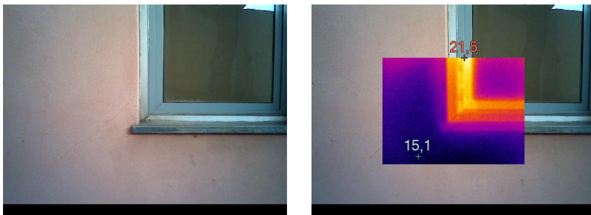
Figura 2.4 – Rilievo termografico dei serramenti
